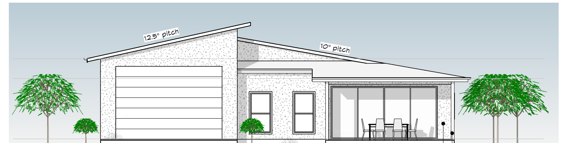
2 Elevation 1 1 : 100
