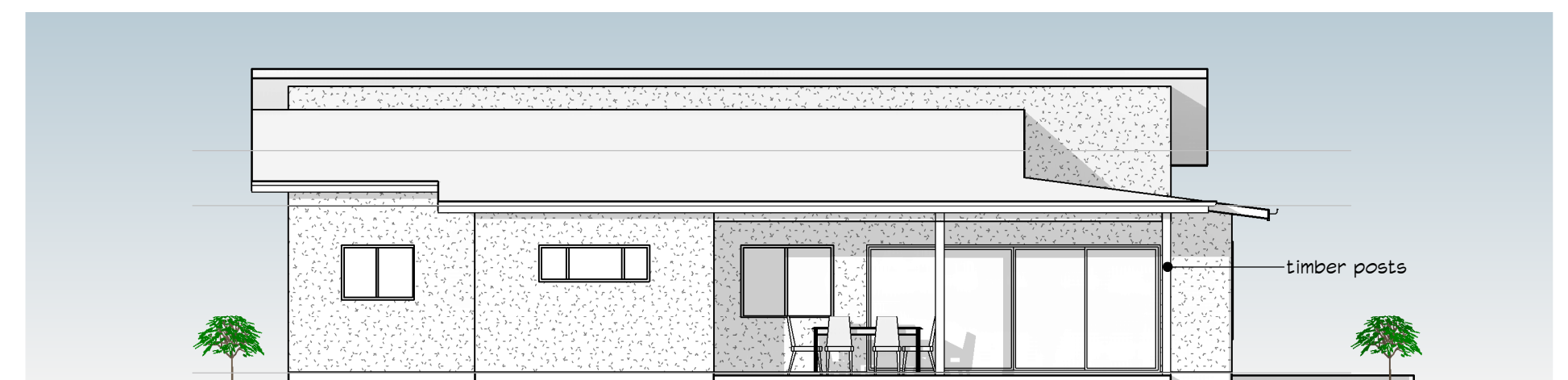
5 Elevation 4 1 : 100
