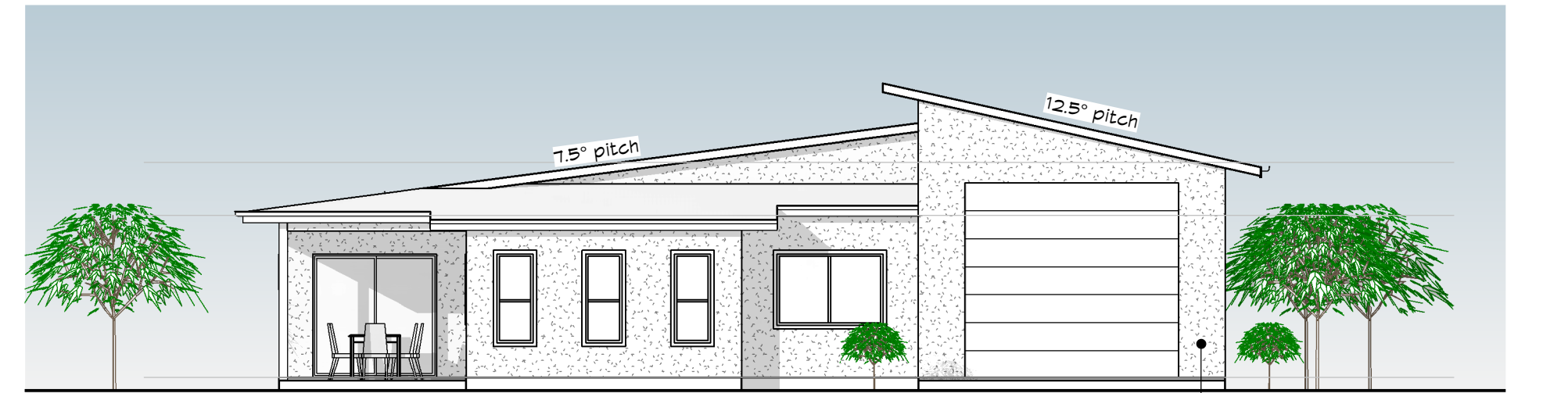
2 Elevation 1 1 : 100
