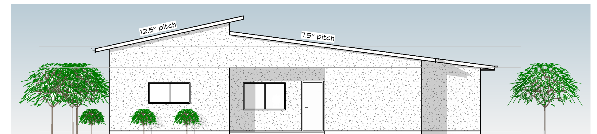
4 Elevation 3 1 : 100
