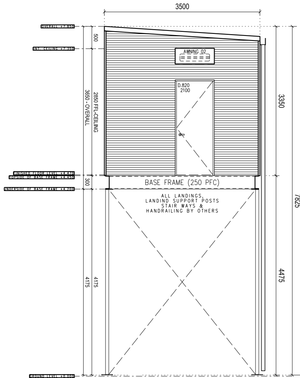
02 - EXTERNAL ELEVATION
