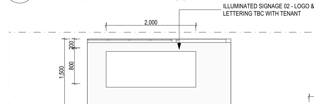
2 SIGNAGE 2 1:50
