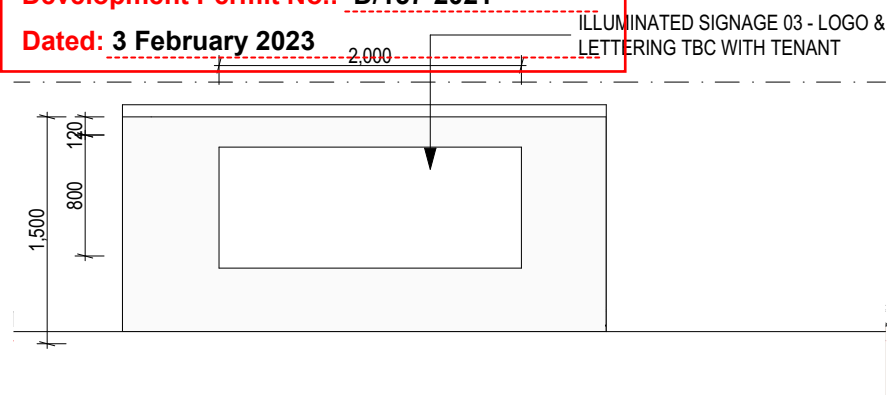
3 SIGNAGE 3 1:50
