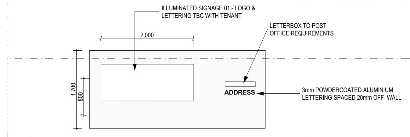
1 SIGNAGE 1 1:50
